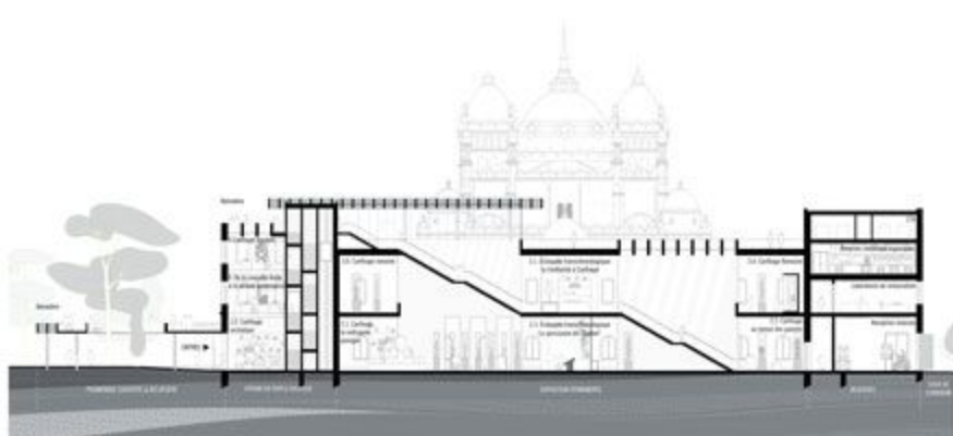
COUPE/ELEVATION DU PARCOURS PERMANENT 1/200
