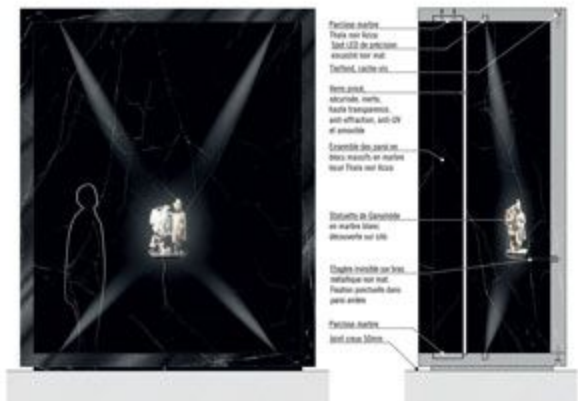
DÉTAIL SCÉNOGRAPHIQUE - GANYMÈDE - ELEVATION/COUPE 1/200
